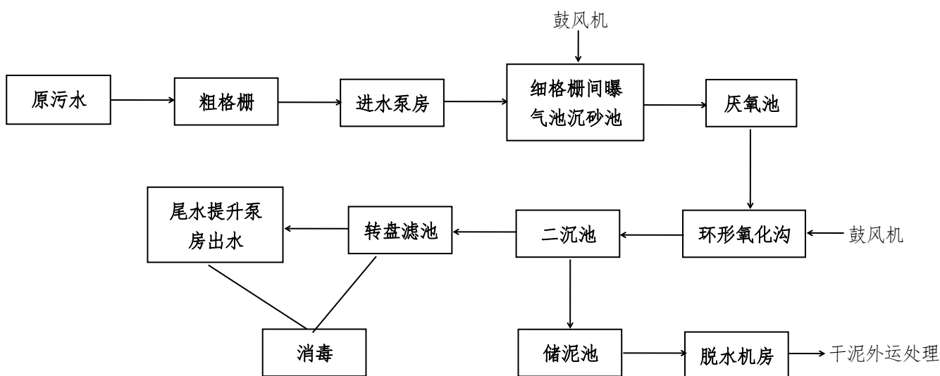
图 2.4-1 拱北水质净化厂三期污水处理工艺流程图
