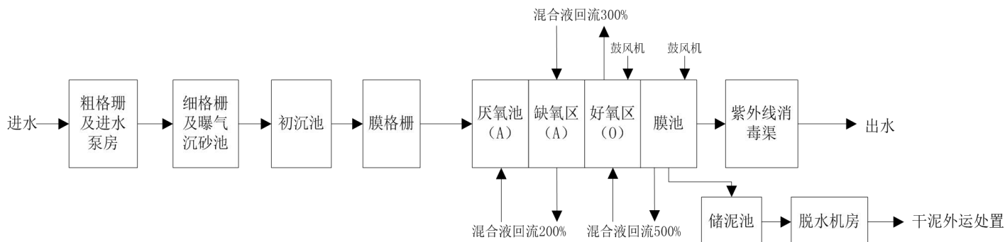
图 2.4-3 拱北水质净化厂扩建工程污水处理工艺流程图
