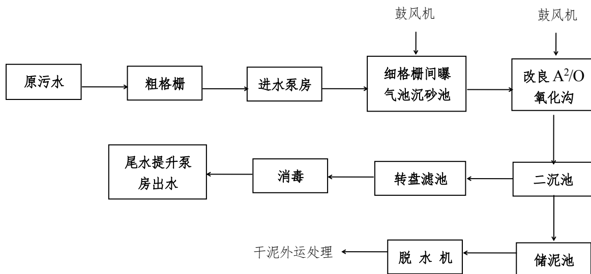
图 2.4-2 拱北水质净化厂改扩一期污水处理工艺流程图
